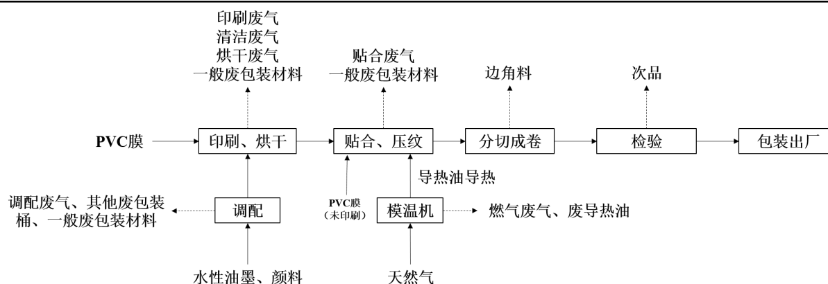
图 2.4-1 待建项目工艺流程及产污环节图
