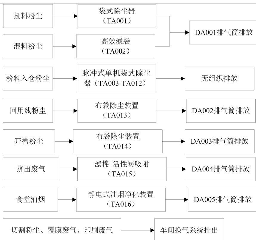
图 4.2-1 项目废气处理系统图
