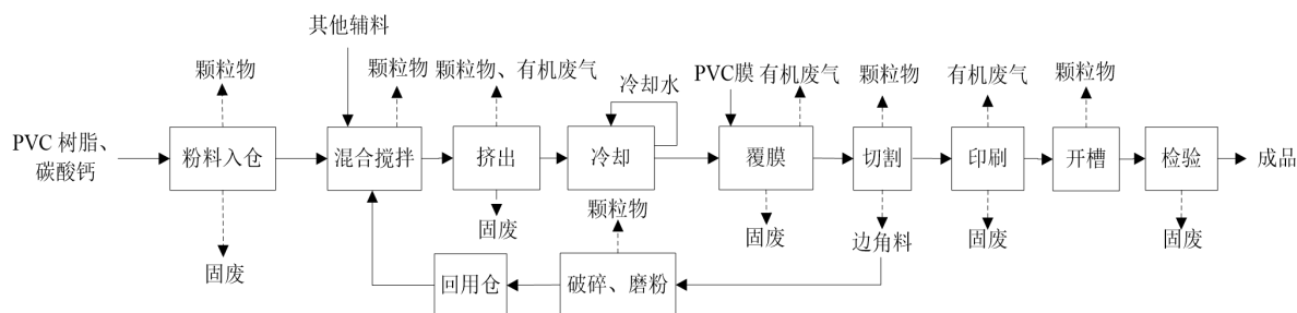
图 2.3-1 环保石塑地板工艺流程及产污环节图
