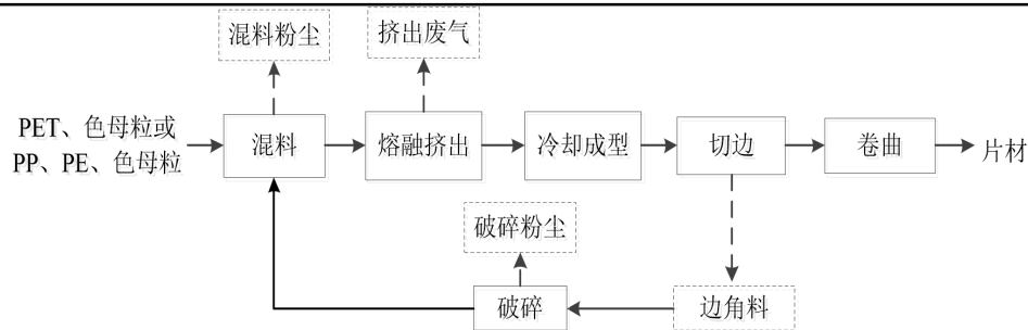
图 2.3-1 片材生产工艺流程及产污环节图
