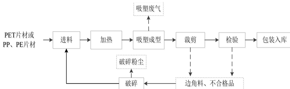
图 2.3-2 食品保鲜容器生产工艺流程及产污环节图
