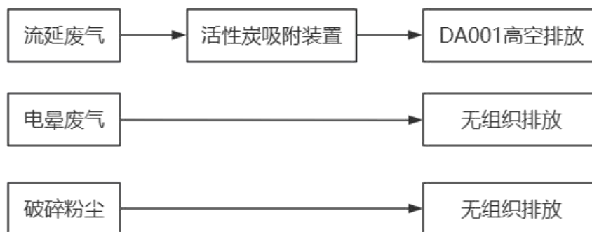
图 3-1 项目废气处理系统图
