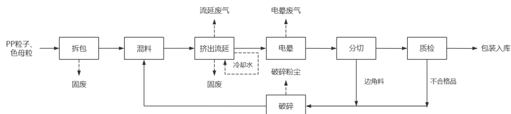
图 2-1 CPP 医用包装膜生产工艺流程图
