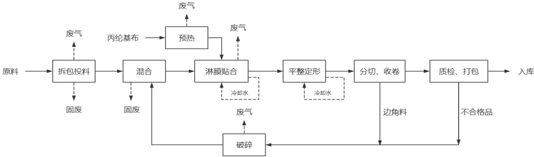
图 2.3-1 生产工艺流程图
